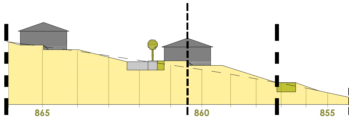
Implantation à l'alignement de la voie de desserte
